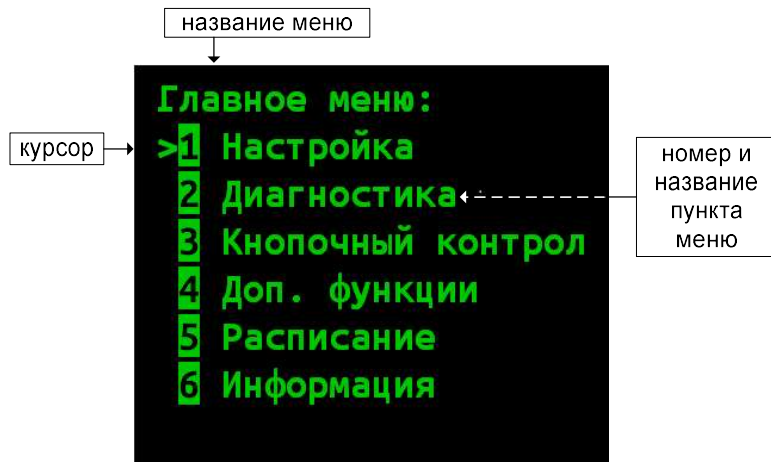
Рисунок 5. Главное меню.
